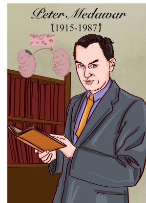
图 7-14 Medawar
