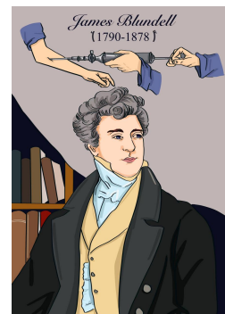
图 7-9 Blundell
