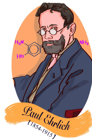
图 7-6 Ehrlich
