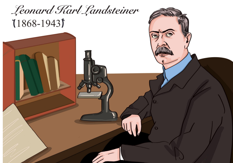
图 7-10 Landsteiner
