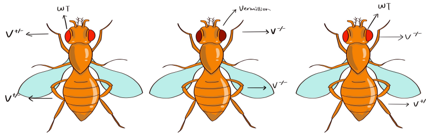
图 4-3 vermilion 嵌合体
