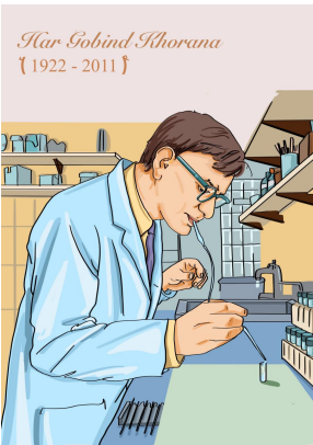
图 4-20 Khorana
