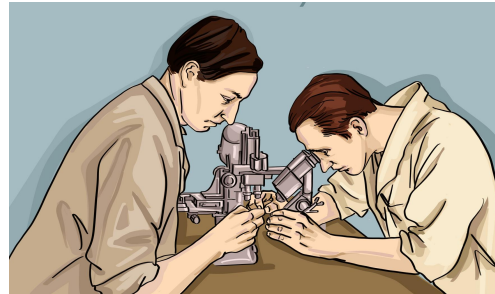
图 4-4 Ephrussi 和 Beadle
