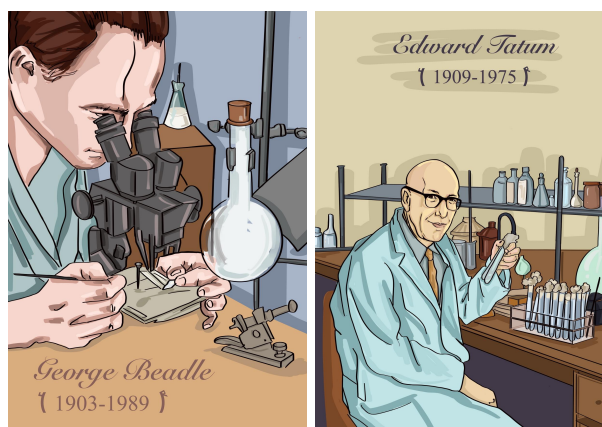
图 4-7 Beadle 和 Tatum
