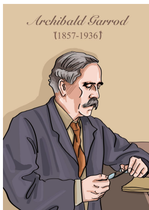
图 4-2 Garrod
